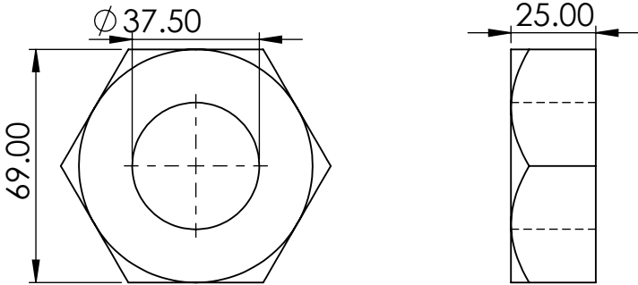
Nut
